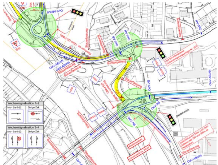
Beispiel Massnahmen Brückenkopf Ost – Kresel Landvogteischloss
