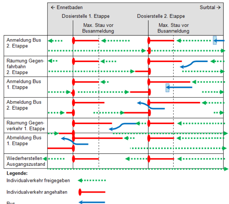
Funktionsschema elektronische Busspur Ehrendingerstrasse
