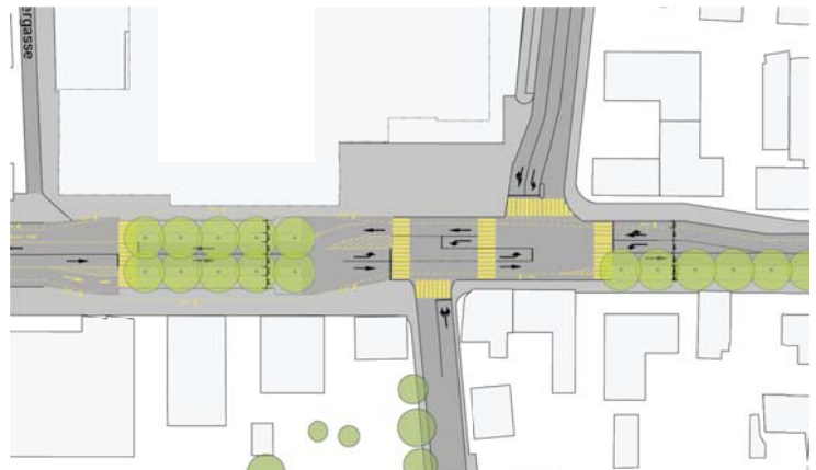
Einer der vorgeschlagenen Umgestaltungsvarianten Knoten Zürcher-/ Emil-Klöti-/ Stationsstrasse.
