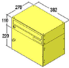
Standard Briefkasten/Depotkasten Typ 27 382 x 110/220 x 270 mm Einwurf 352 x 33 mm
