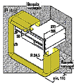
RS4100 Teilwandeinbau
