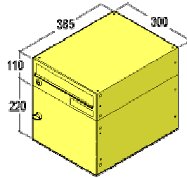
Standard Briefkasten/Depotkasten Typ 38 300 x 110/220 x 385 mm Einwurf 262 x 33 mm
