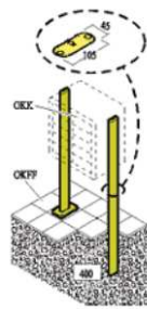
ALU-Ovalrohrständer, 105 x 45 mm
