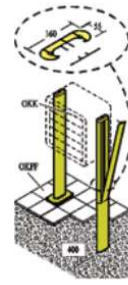
ALU-Ovalrohrständer, 160 x 55 mm
