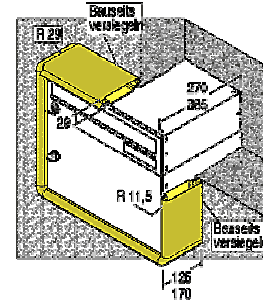
RS2000 Teilwandeinbau
