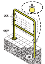
Stahl-Rundrohrgestell Ø 60mm preisgünstige Alternative: nur seitliche Ständer
