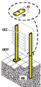
ALU-Ovalrohrständer, 105 x 45 mm
